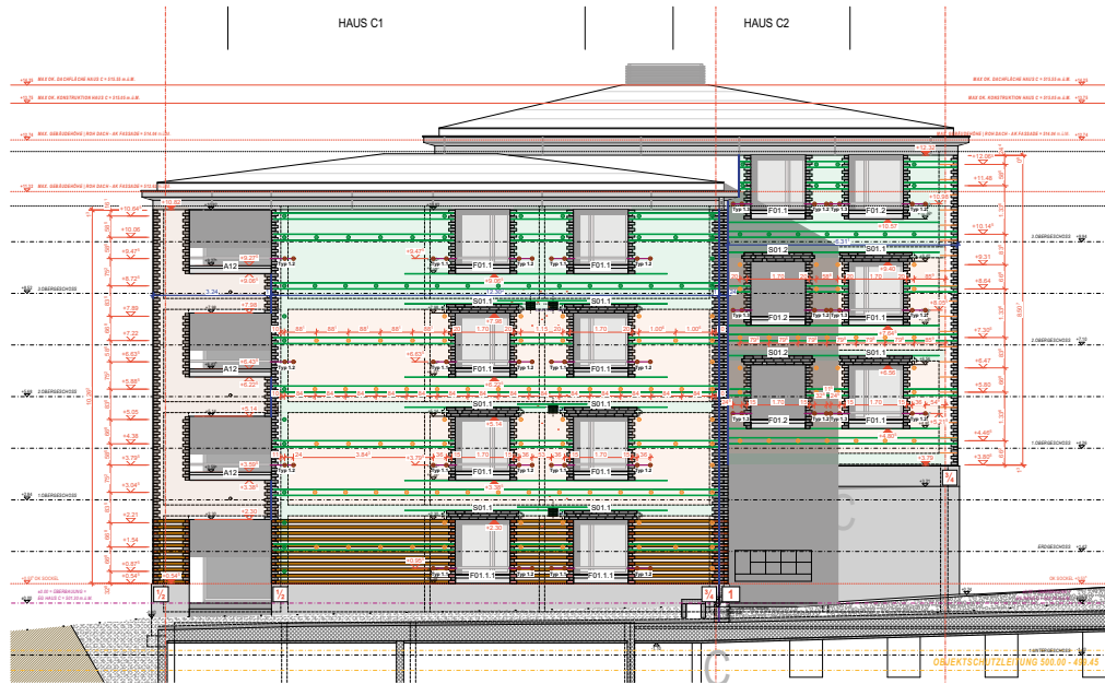
Ost-Fassade
