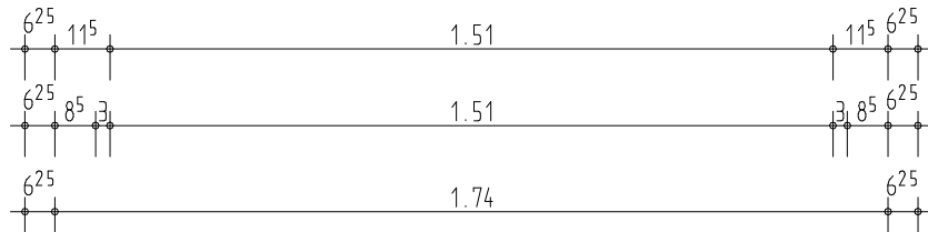
Draufsicht
