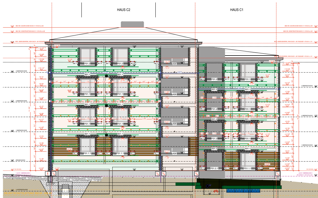
West-Fassade
