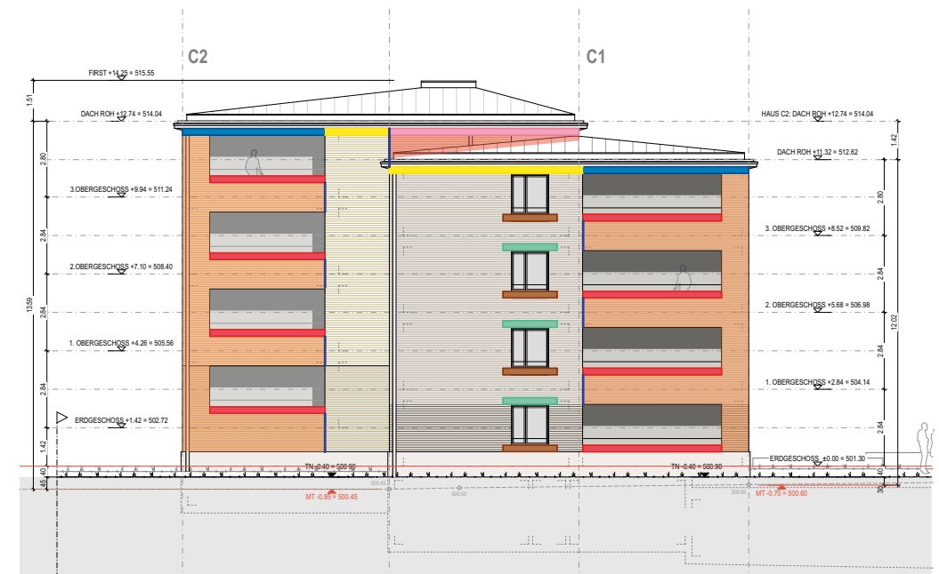
Südwest-Fassade
