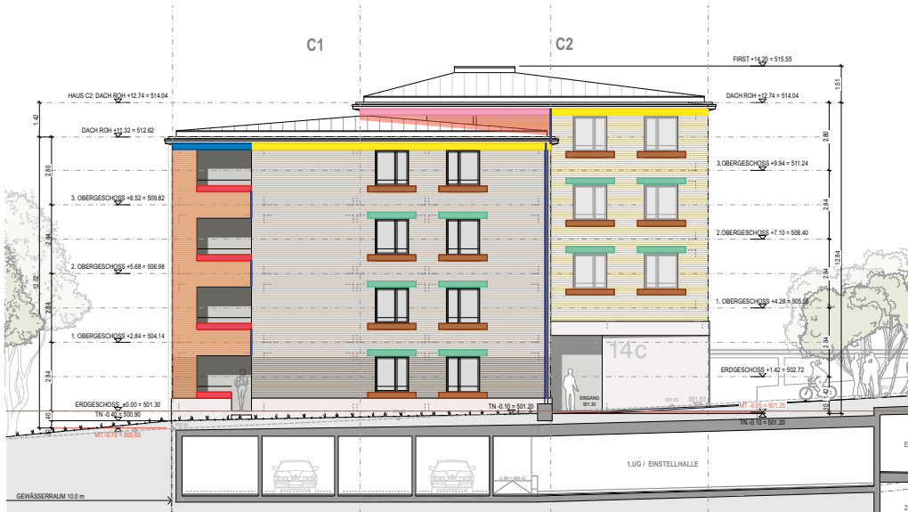
Südost-Fassade
