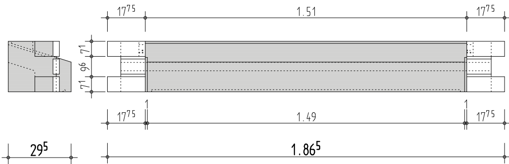
Ansicht
